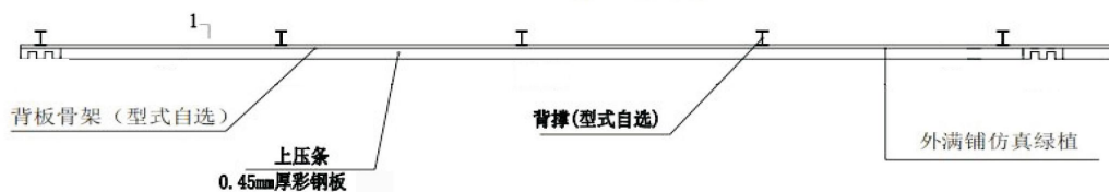
仿真绿植围墙俯视图
