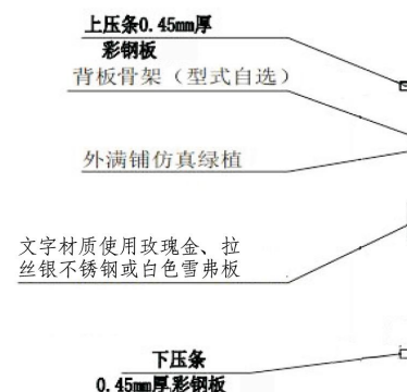
仿真绿植1-1剖面图
