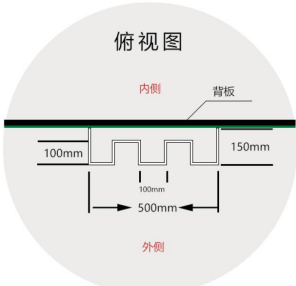
装饰柱节点图
