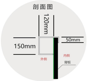
上压条节点图
