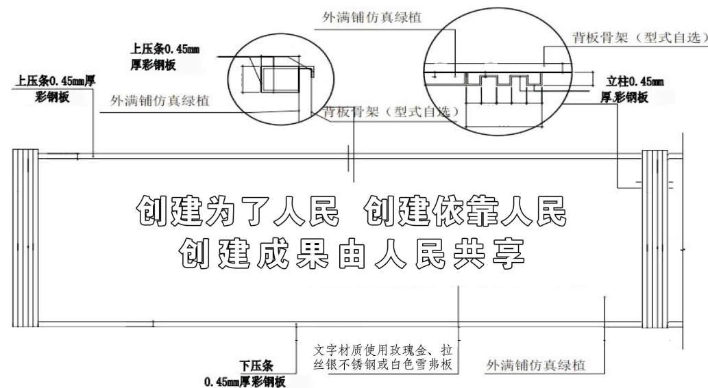
仿真绿植围墙正视图
